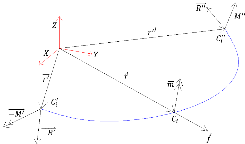
Figura 16.6 - Esforços externos e internos em um elemento infinitesimal de barra
