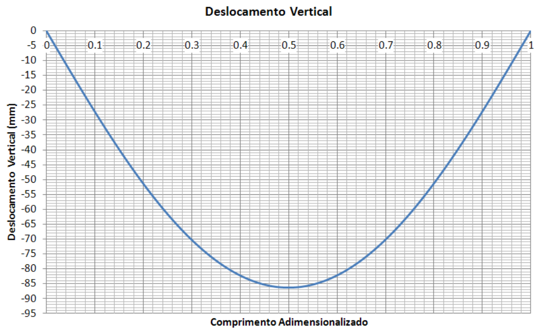
Figura 4.20 – Deslocamento Vertical no modelo. Com peso próprio
