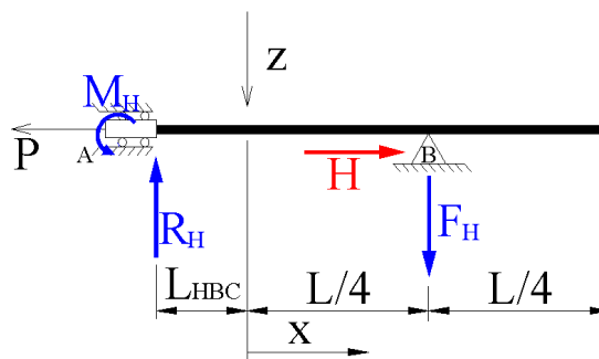
Figura 12.11 - Modelo simplificado
