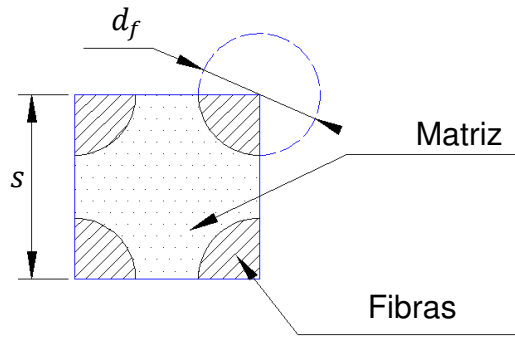
Figura 6.8 – Representação idealizada de disposição de fibras de seções circulares em arranjos quadrados.
