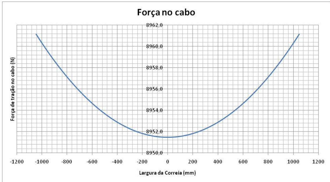
Gráfico 7.1 - Força no cabo de aço em função da posição relativa ao centro da correia
