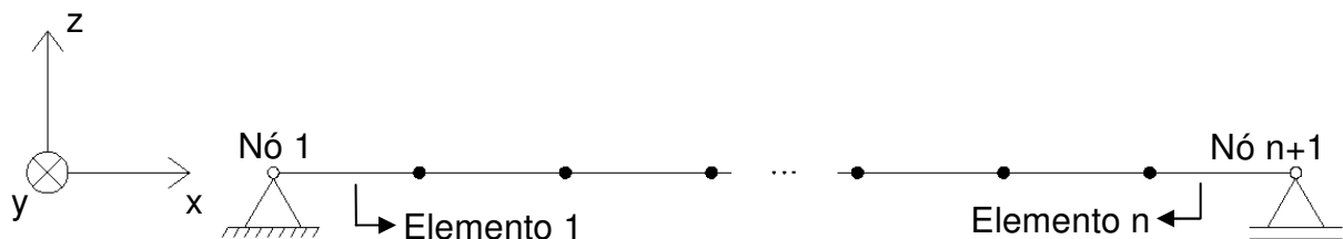
Figura 4.17 - Modelo utilizado para a correia
