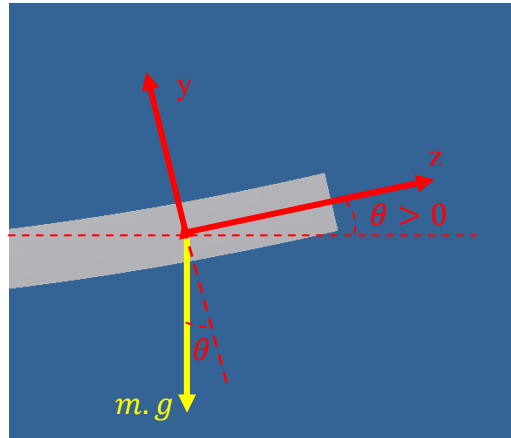
Figura 4.16 - Carregamento por unidade de comprimento mg
