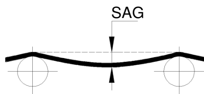
Figura 4.6 - SAG entre roletes do transportador
