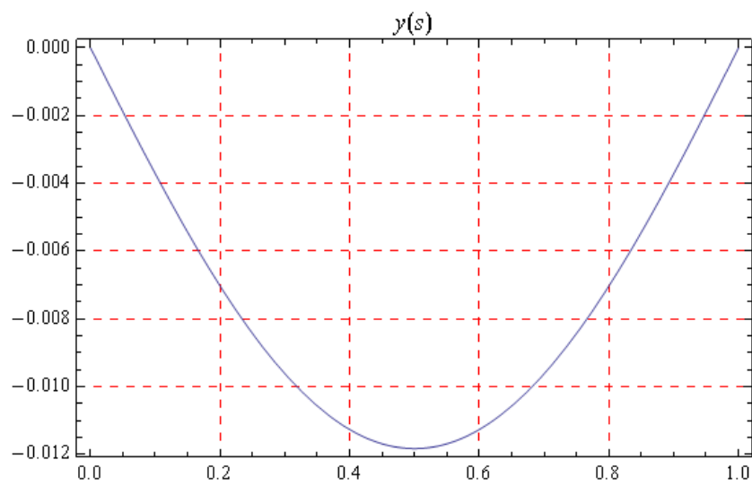
Gráfico 4.7- Deslocamento Vertical x Curvatura Adimensionalizada.
