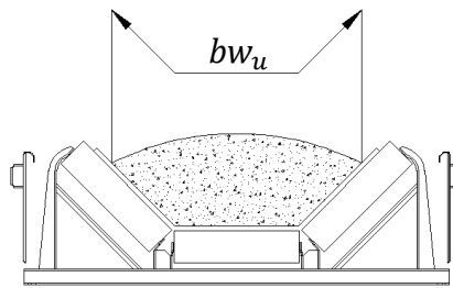
Figura 10.3: Largura da correia útil.
