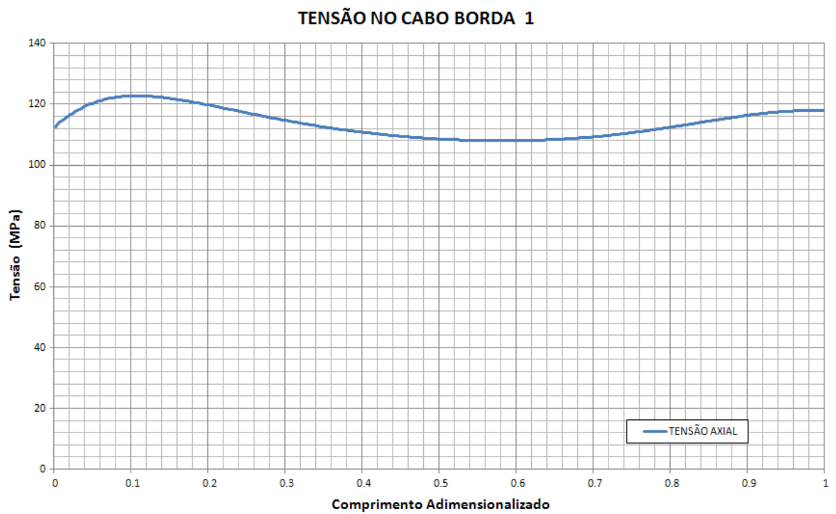
Figura 5.16 - Tensão no ponto médio da seção transversal do cabo de aço de um dos lados da correia.
