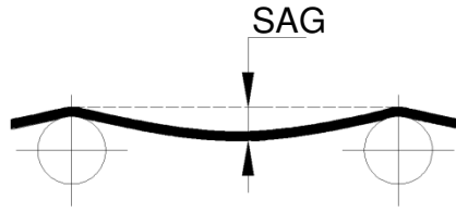
Figura 3.2 - SAG entre roletes do transportador.
