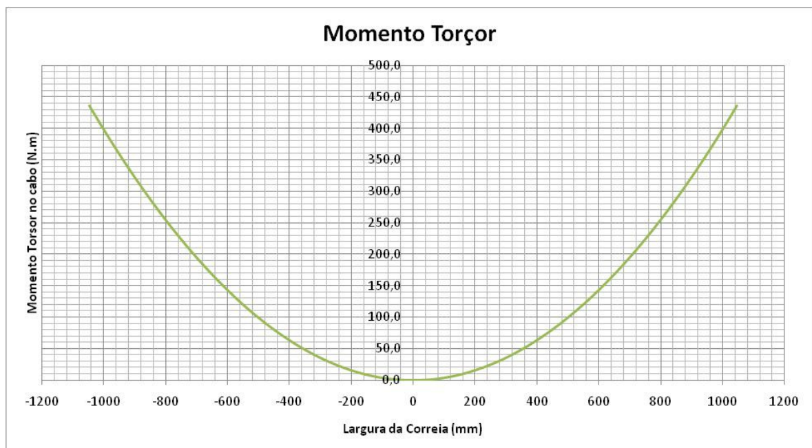
Gráfico 7.2 – Momento Torçor no cabo de aço em função da posição relativa ao centro da correia
