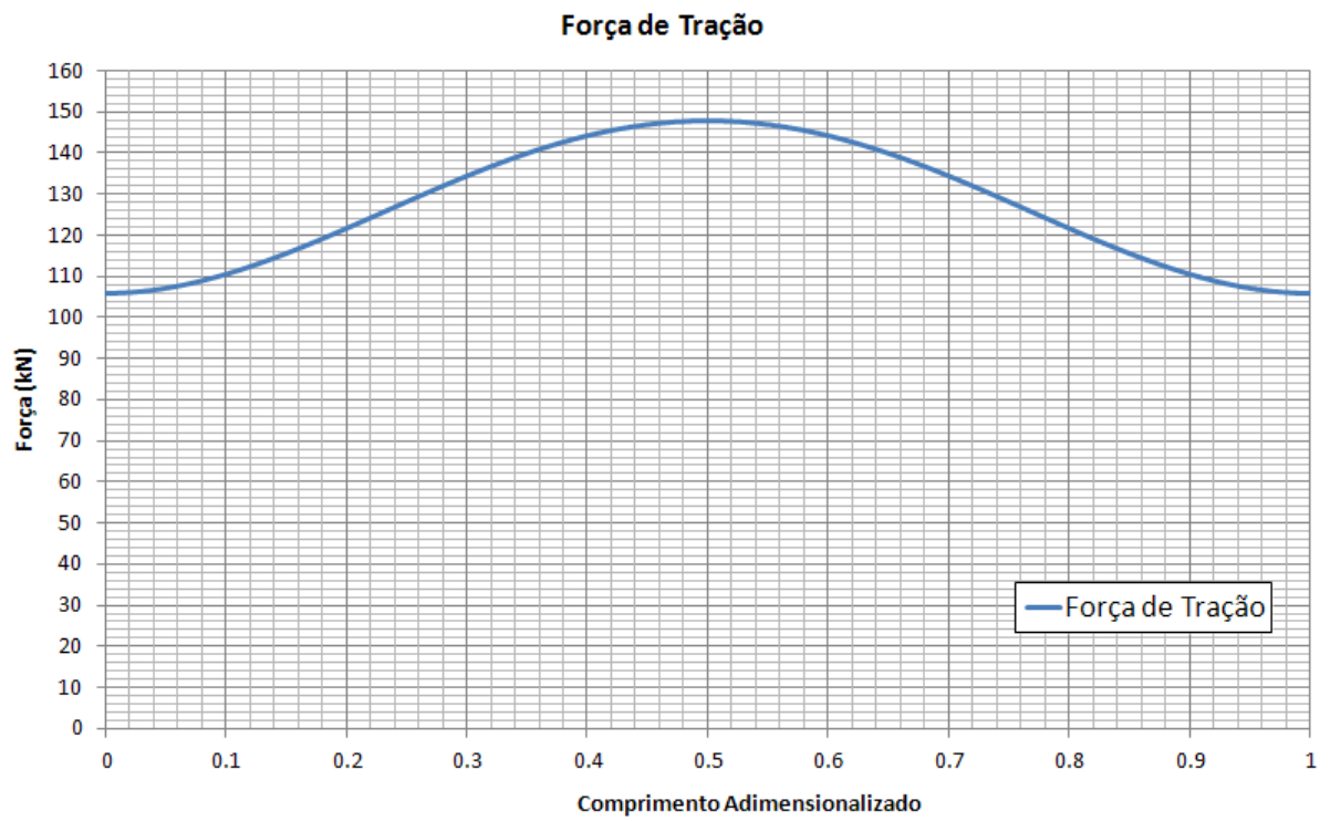
Figura 4.19 - Força de tração no modelo. Com peso próprio
