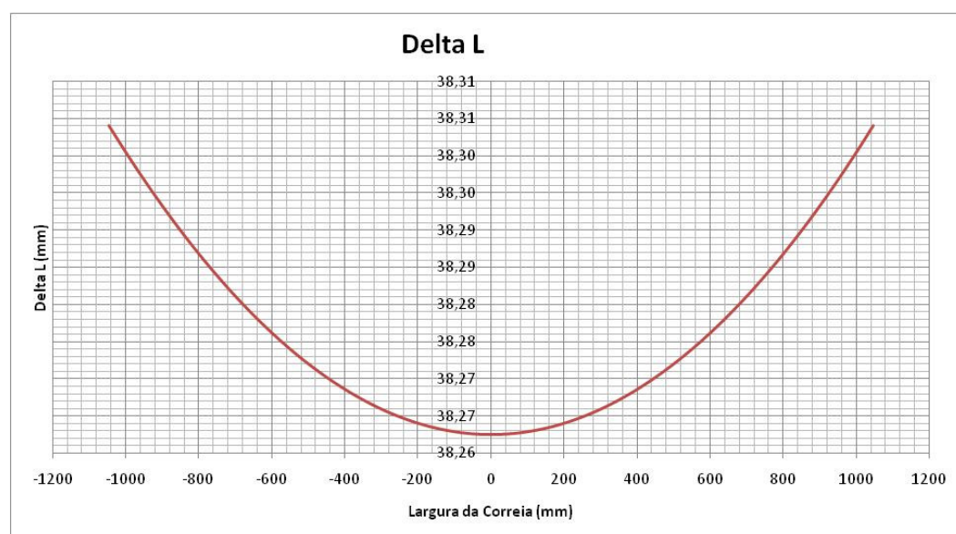
Gráfico 7.4 – Variação no comprimento do cabo de aço em função da posição relativa ao centro da correia
