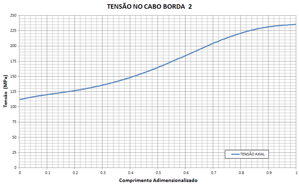
Figura 5.18 - Tensão no ponto médio da seção transversal do cabo de aço do outro lado da correia.
