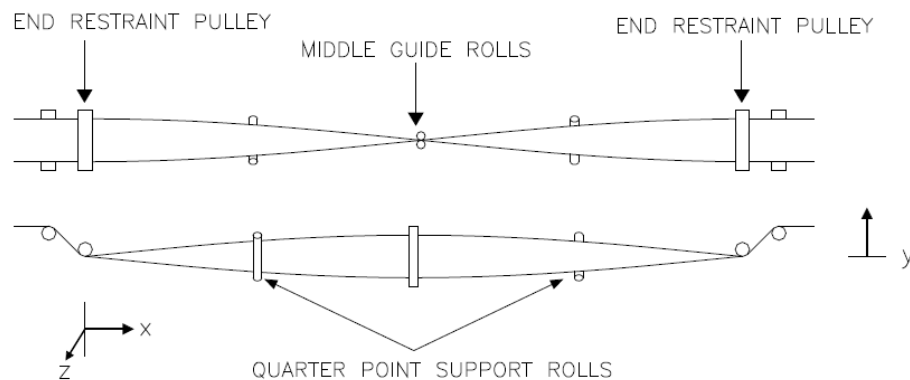
Figura 2.5 - Posição dos pontos intermediários. LEMMON, 2002
