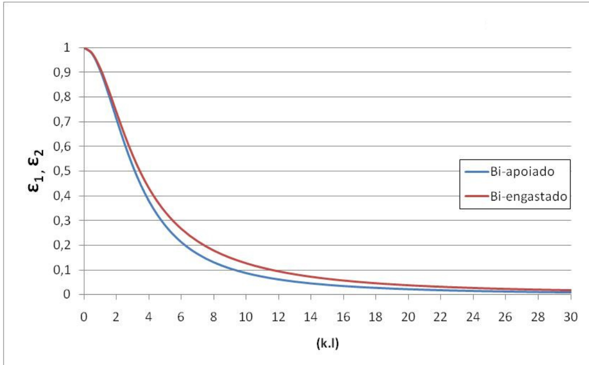
Figura 4.13 - Comparação entre modelos bi-apoiado e bi-engastado
