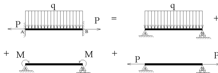
Figura 4.11 - Decomposição do modelo hiperestático em modelos isostáticos fundamentais
