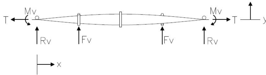
Figura 12.2 - Forças no plano vertical. LEMMON, 2002
