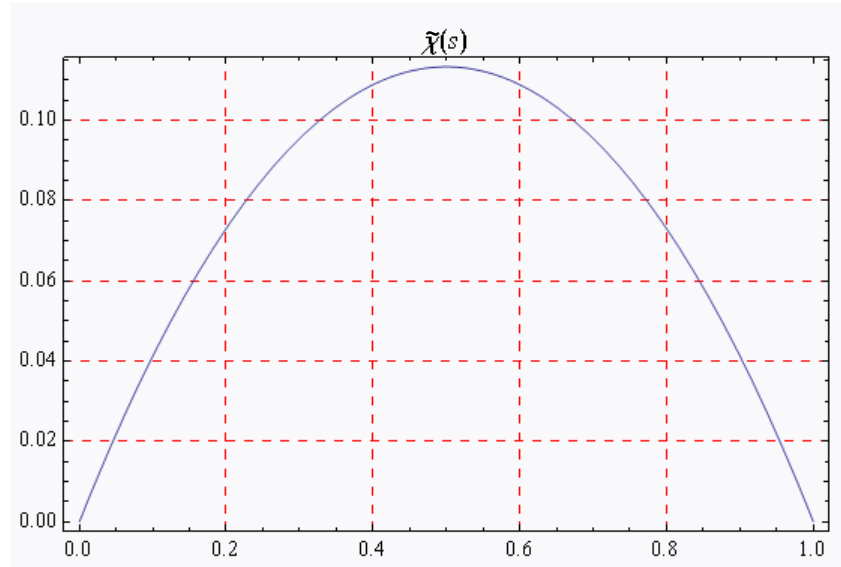
Gráfico 4.6 - Curvatura x Coordenada Curvilínea. Ambos adimensionalizados.
