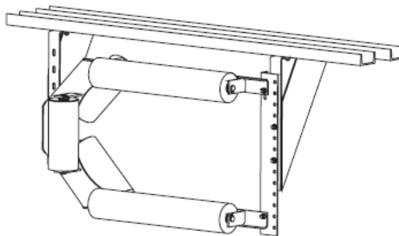
Figura 2.4 – Belt Turning Sandvik.
