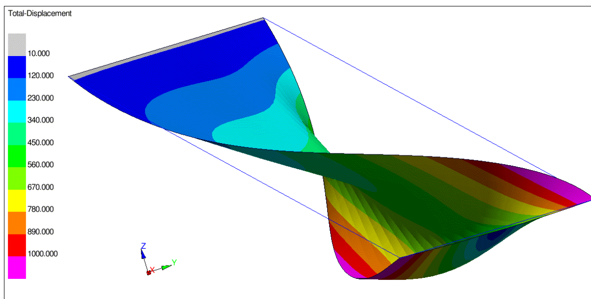
Figura 5.19- Deslocamento total dos elementos
