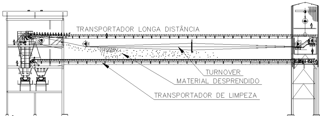
Figura 10.2: Turnover na região de descarga e transportador de limpeza.
