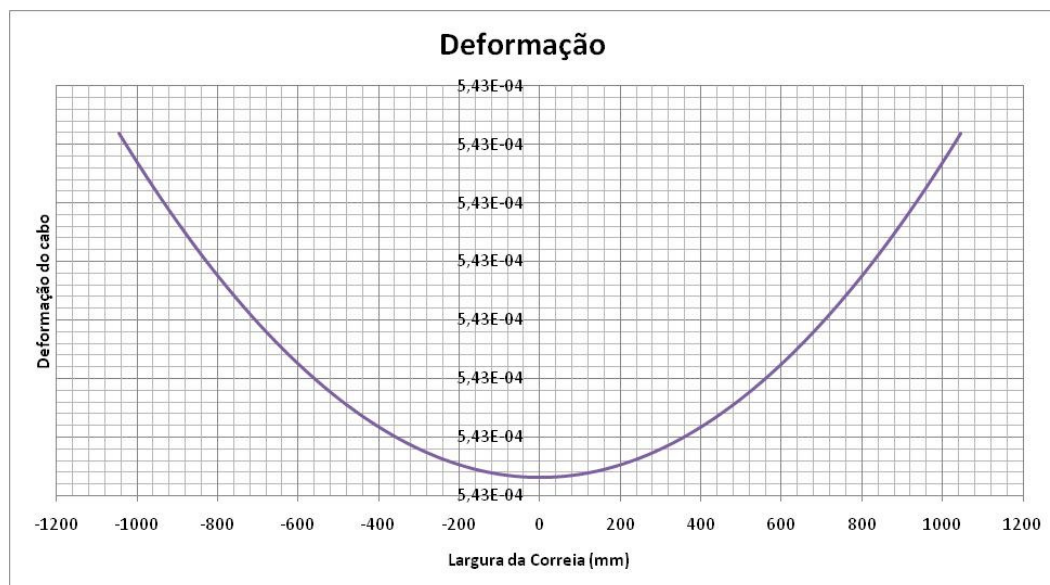
Gráfico 7.3 – Deformação no cabo de aço em função da posição relativa ao centro da correia
