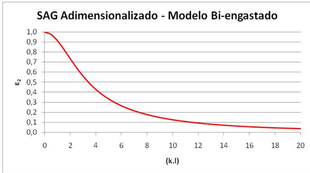
Figura 4.12 - SAG Adimensionalizado - Modelo Bi-engastado
