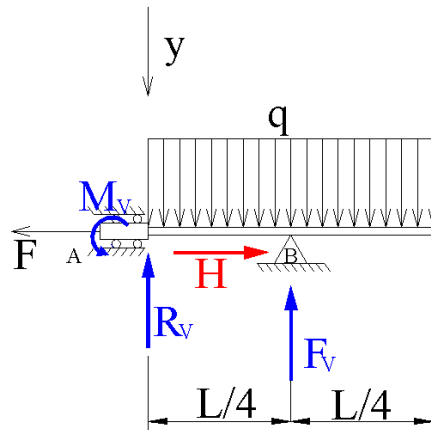
Figura 12.5 - Modelo simplificado
