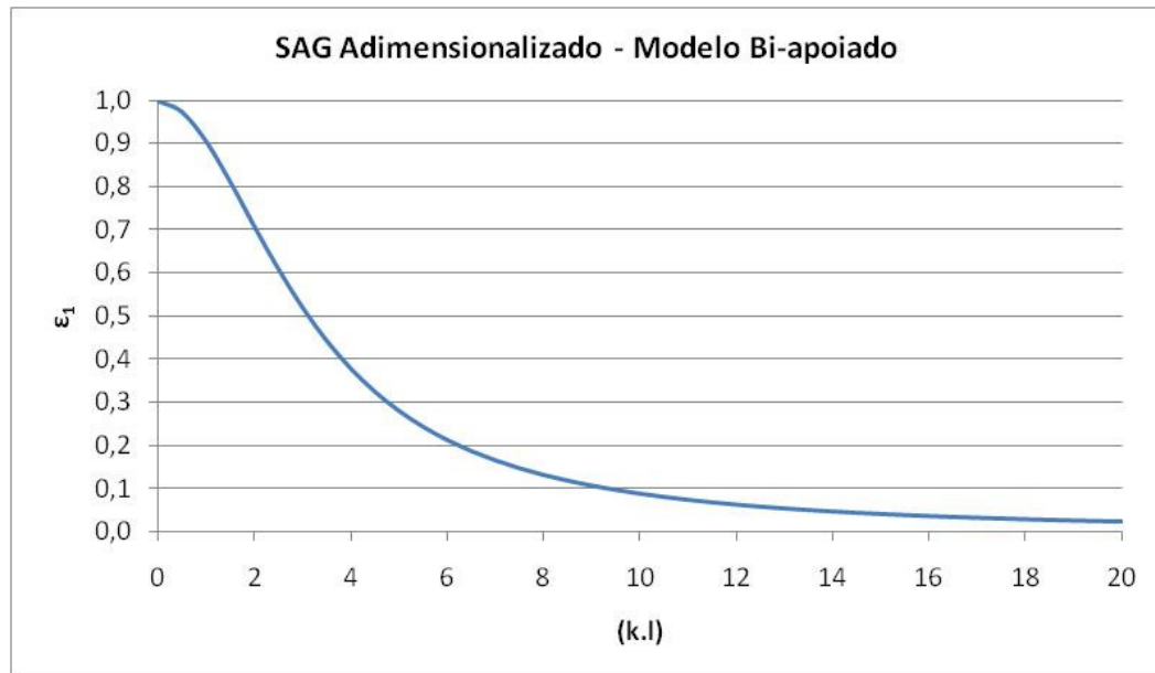
Figura 4.5 - SAG Adimensionalizado - Modelo bi-apoiado
