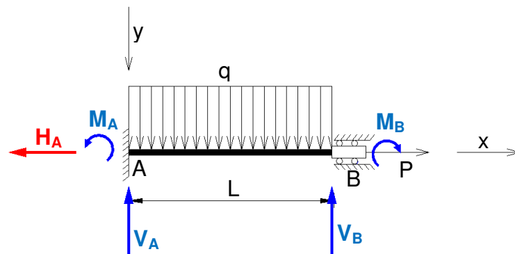
Figura 4.9 - Reações de apoio
