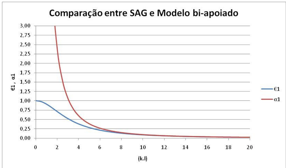
Gráfico 4.1 - Comparação entre SAG e Modelo bi-apoiado. Para 0 \leq k.l \leq 20 .
