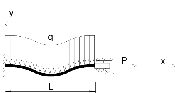
Figura 4.8 - Configuração deformada
