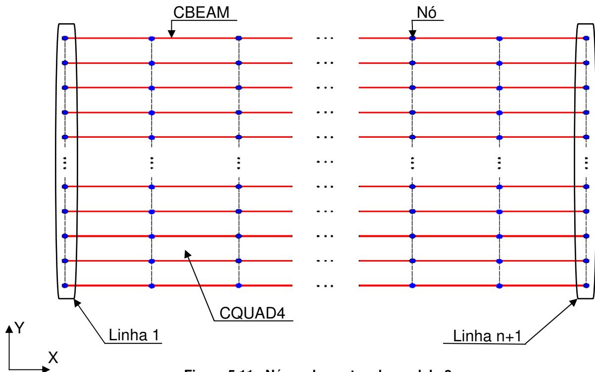
Figura 5.11 - Nós e elementos do modelo 2
