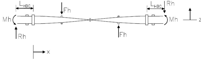
Figura 12.8- Forças no plano horizontal. LEMMON, 2002
