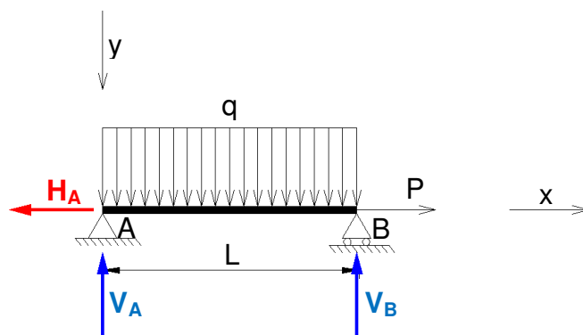
Figura 4.3 - Reações de apoio
