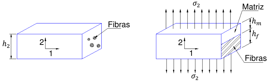
Figura 6.6 - Modelo para obtenção de propriedades transversais dos materiais compostos unidirecionais.
