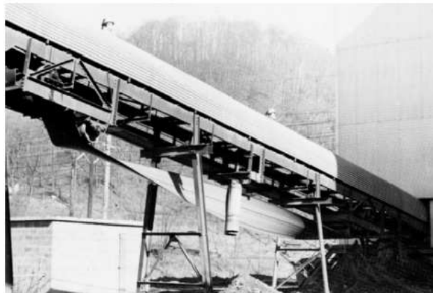
Figura 2.1 – Visão de uma correia em giro de 180°. (Mercúrio)
