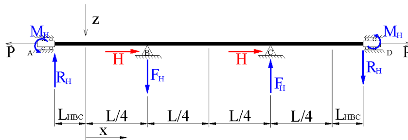
Figura 12.10 - Reações de Apoio
