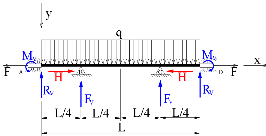
Figura 12.3 - Modelo Adotado
