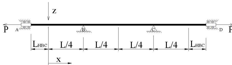
Figura 12.9 - Modelo Adotado
