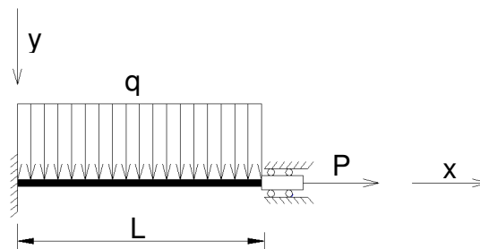
Figura 4.7 - Modelo adotado
