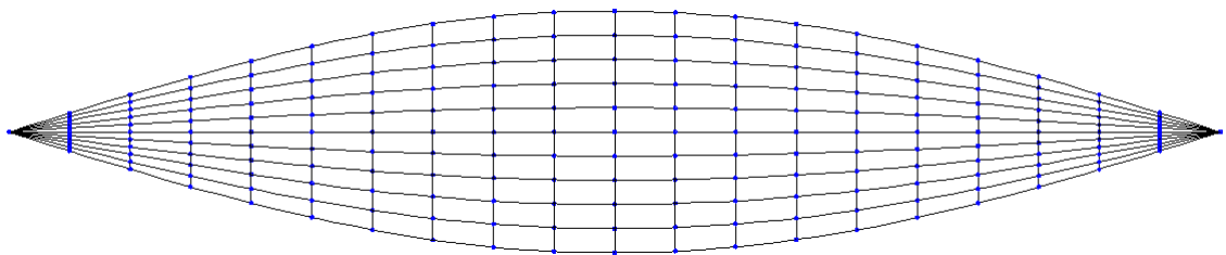
Figura 5.9 – Vista frontal da correia – Configuração deformada
