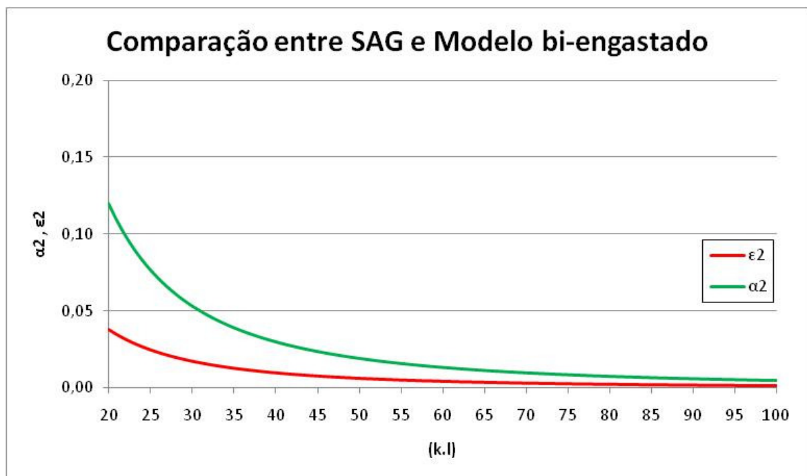
Gráfico 4.4 - Comparação entre SAG e Modelo bi-engastado. Para 20 \leq k.l \leq 100 .
