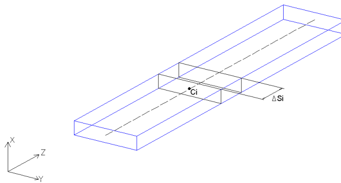
Figura 16.1 - Configuração não-deformada
