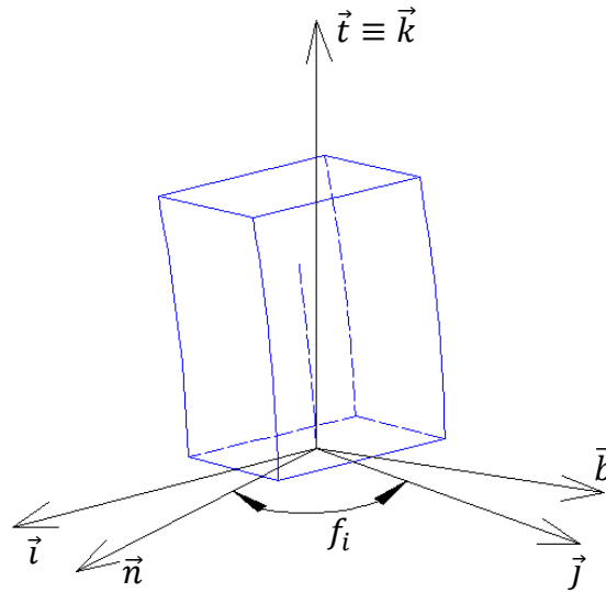
Figura 16.3 - Detalhe do eixo central na configuração deformada
