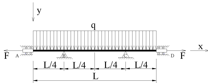
Figura 12.3 - Modelo Adotado
