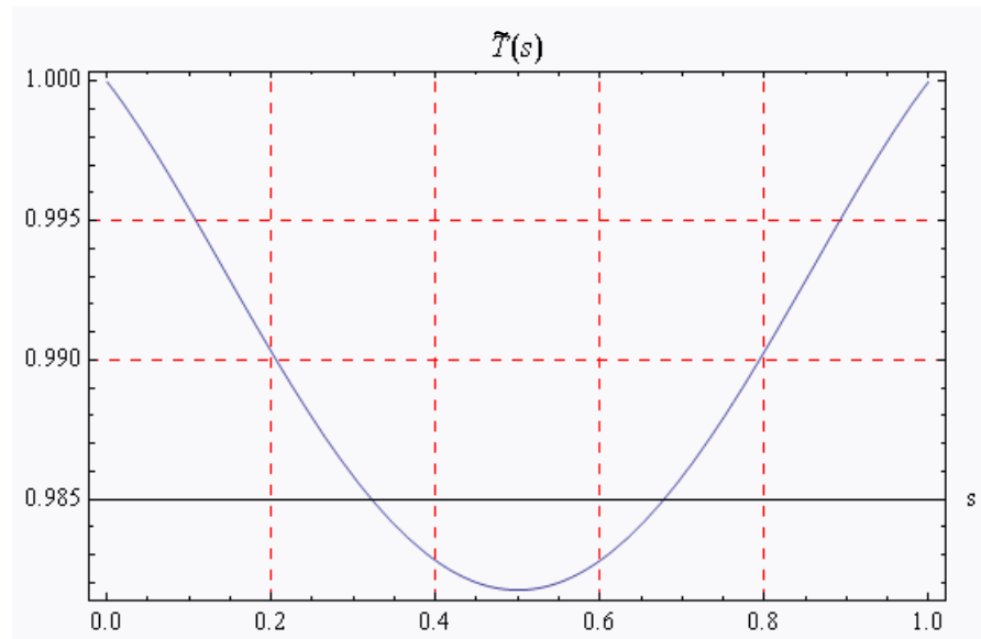
Gráfico 4.8 - Esforço de Tração x Coordenada Curvilínea. Ambos adimensionalizados.
