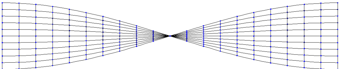
Figura 5.10 – Vista superior da correia – Configuração deformada
