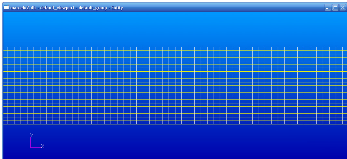
Figura 5.13 - Malha do modelo em MSC Patran. (Ampliação)
