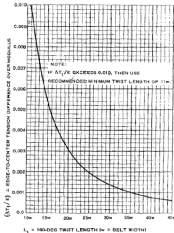
Figura 3.1 - Figura apresentada para determinar o comprimento do turnover. (Goodyear, 1975)
