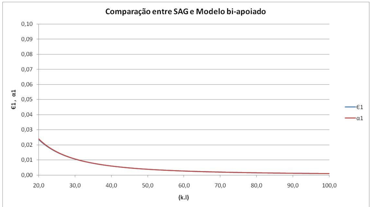
Gráfico 4.2 - Comparação entre SAG e Modelo bi-apoiado. Para 20 \leq k.L \leq 100 .
