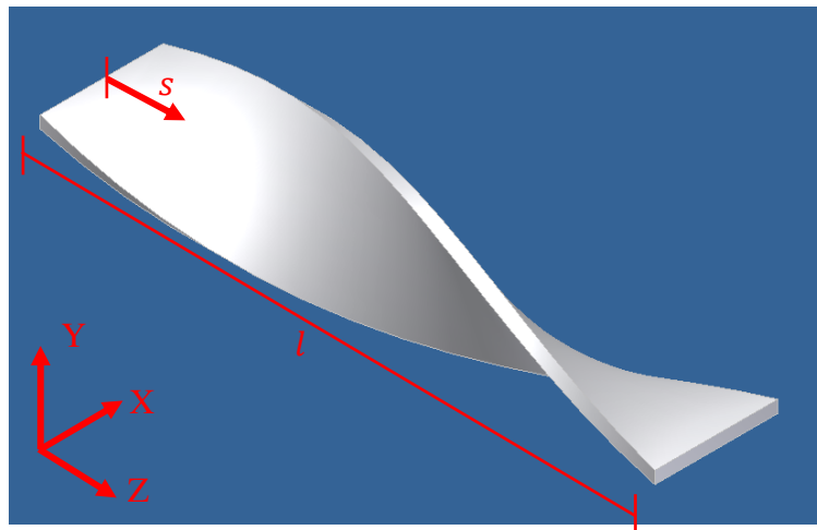
Figura 5.6 - Comprimento do virador e definição de s
