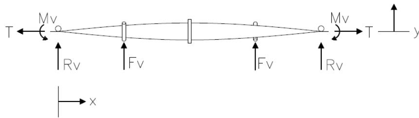
Figura 3.4 - Diagrama de esforços - Plano Vertical. (LEMMON, 2002)
