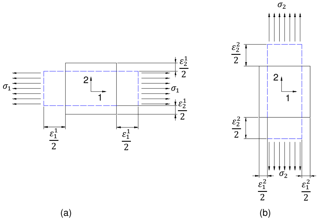
Figura 6.3 – Tensões e deformações normais nas direções 1 e 2
