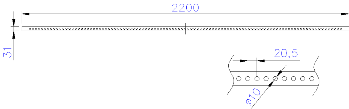
Figura 7.1 - Seção transversal da correia – Dimensões em milímetros
