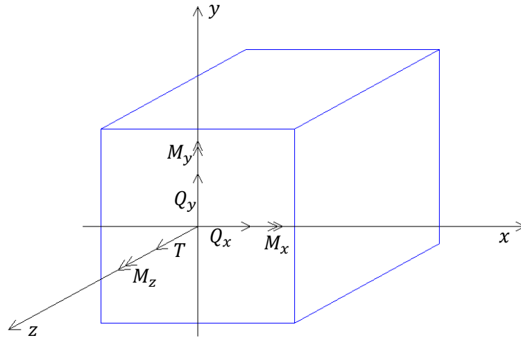
Figura 16.4 - Esforços solicitantes em uma seção genérica da barra
