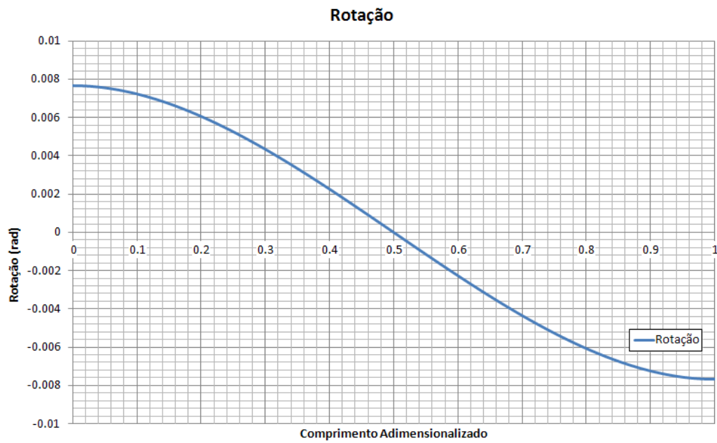
Figura 4.21 – Rotação no modelo. Com peso próprio
