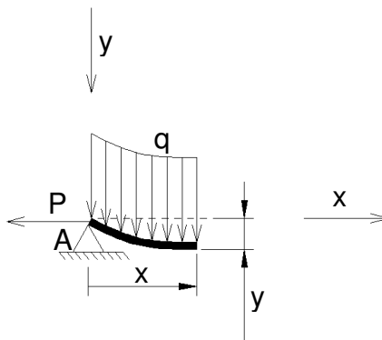
Figura 4.2- Configuração deformada
