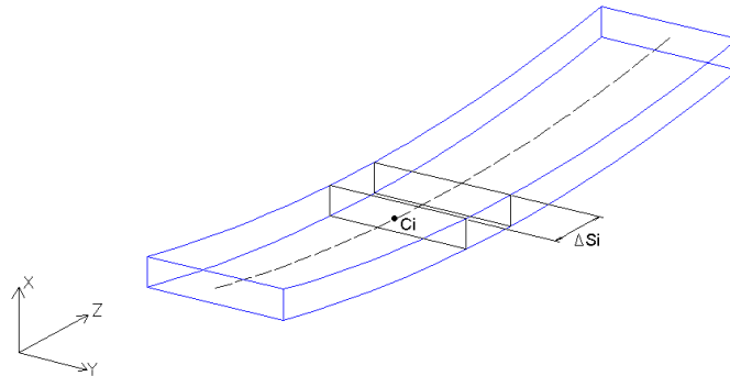
Figura 16.2 - Configuração deformada
