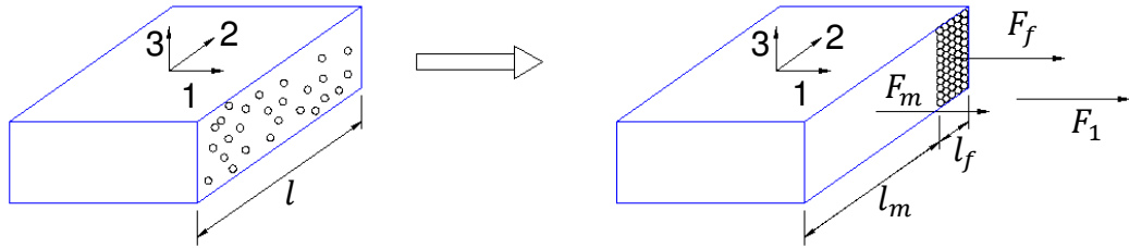
Figura 6.5 - Forças suportadas pelas fibras, F_f , pela matriz, F_m e pelo composto, F_1
