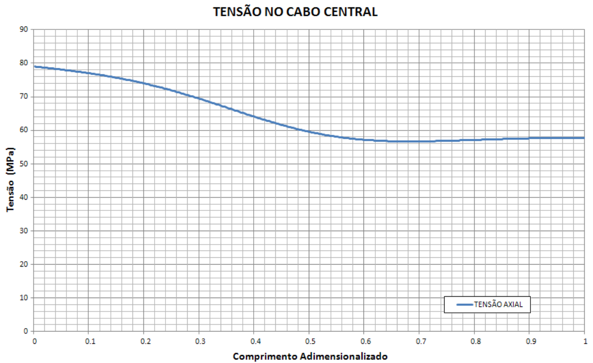
Figura 5.17- Tensão no ponto médio da seção transversal do cabo de aço central da correia.
