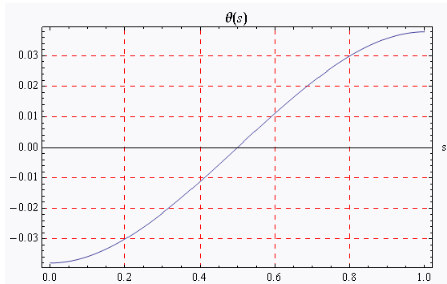
Gráfico 4.5- Rotação x Coordenada Curvilínea. Ambos adimensionalizados.
