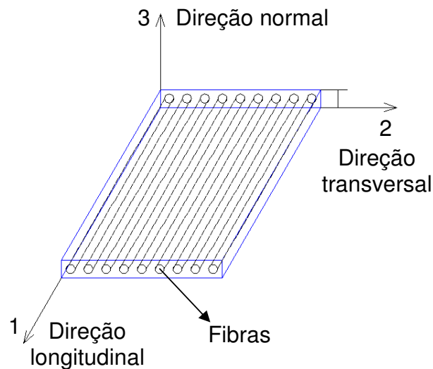
Figura 6.2 – Direções principais de propriedades mecânicas em uma lâmina
