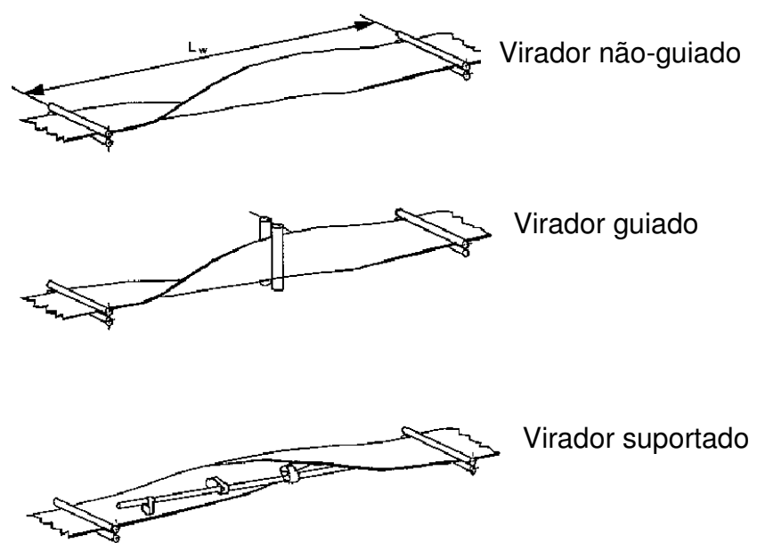
Figura 2.6 – Variedade construtiva de viradores. (DIN 22101).
