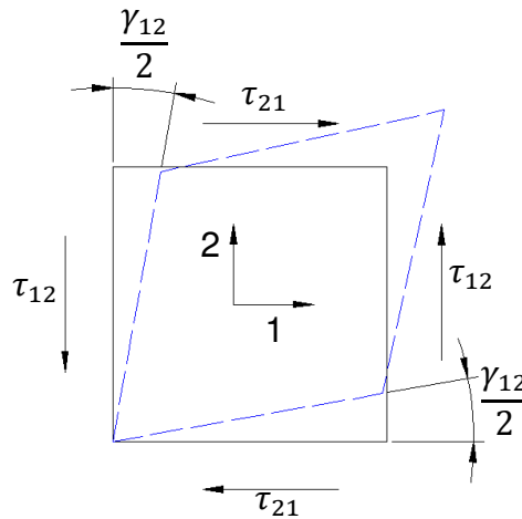
Figura 6.4 - Tensão e deformação cisalhante
