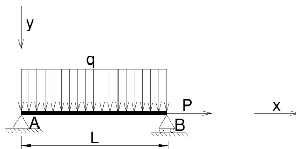
Figura 4.1 - Modelo adotado
