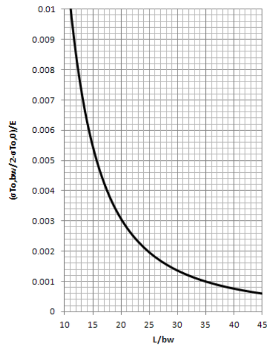
Gráfico 3.2 - Subtração da tensão de borda e tensão de centro em função do comprimento do virador adimensionalizado
