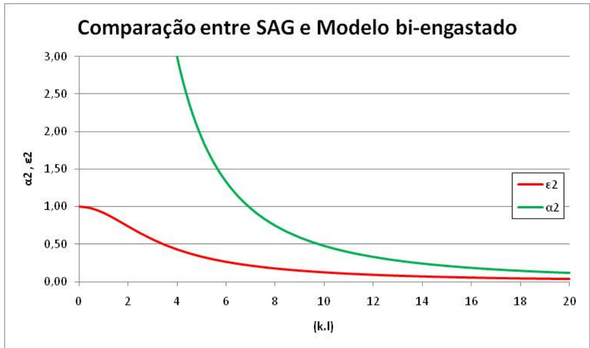
Gráfico 4.3 - Comparação entre SAG e Modelo bi-engastado. Para 0 \leq k.l \leq 20 .
