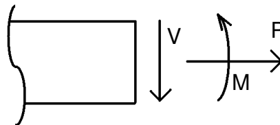
Figura 4.4 - Esforços na seção de corte
