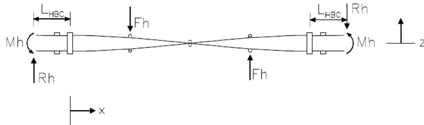
Figura 3.5 - Diagrama de esforços - Plano Horizontal. (LEMMON, 2002)
