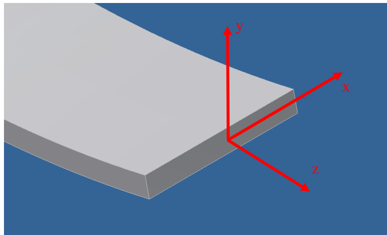
Figura 4.15 - Eixos locais de flexão (x,y) e torção (z) da correia
