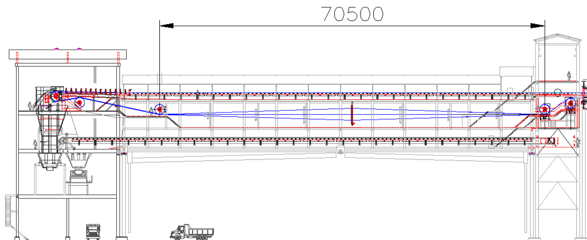
Figura 7.2 - Turnover em estudo - Dimensão em milímetros
